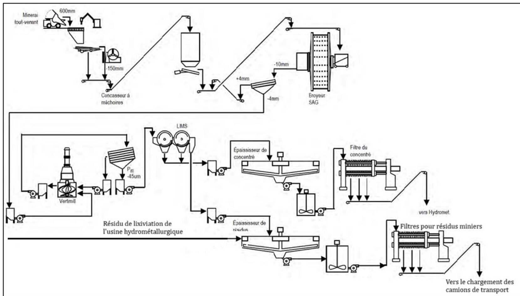
Figure 17.1 – Schéma de procédé simplifié
