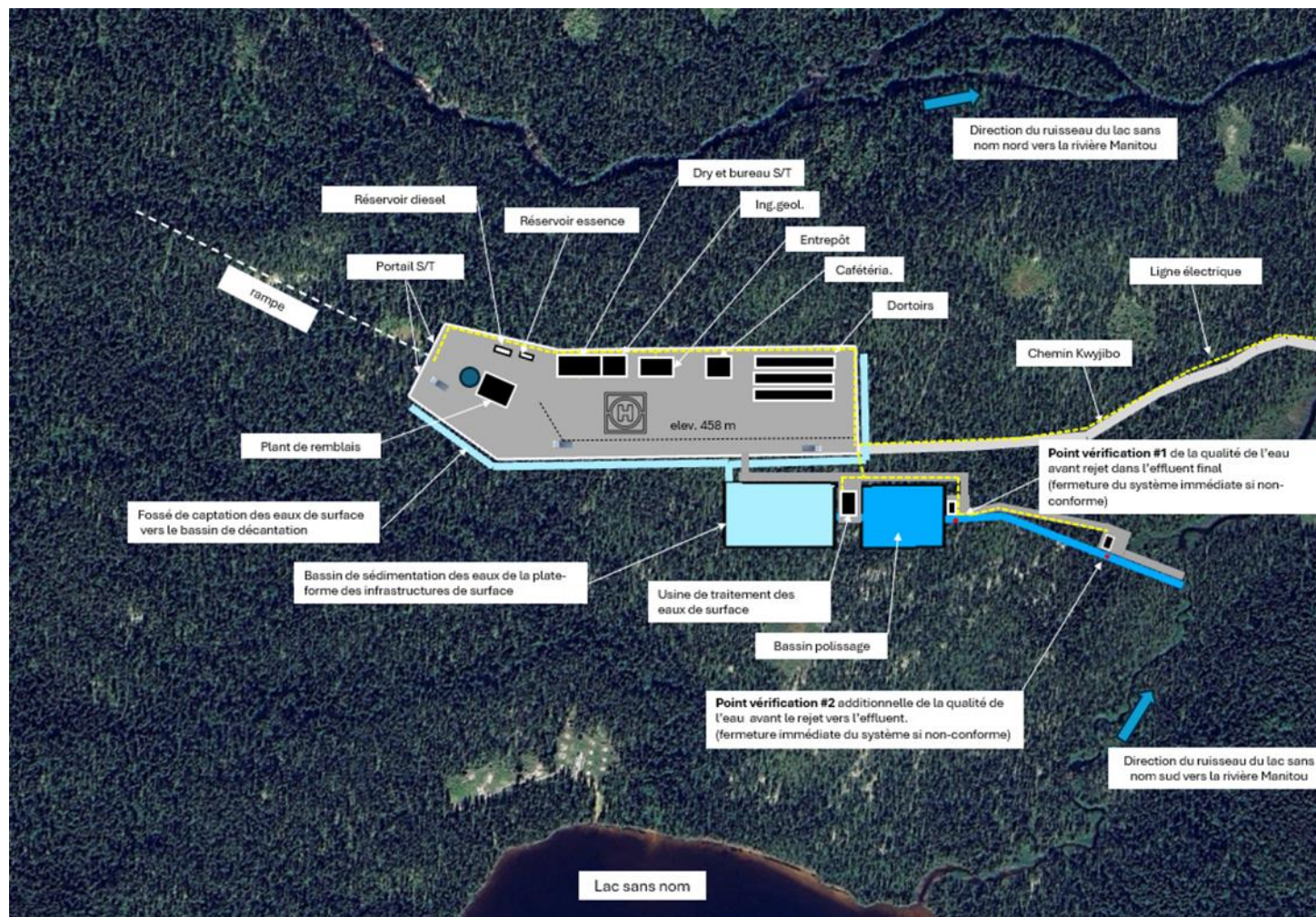
Figure 18.1 – Arrangement général - site de Kwyjibo
