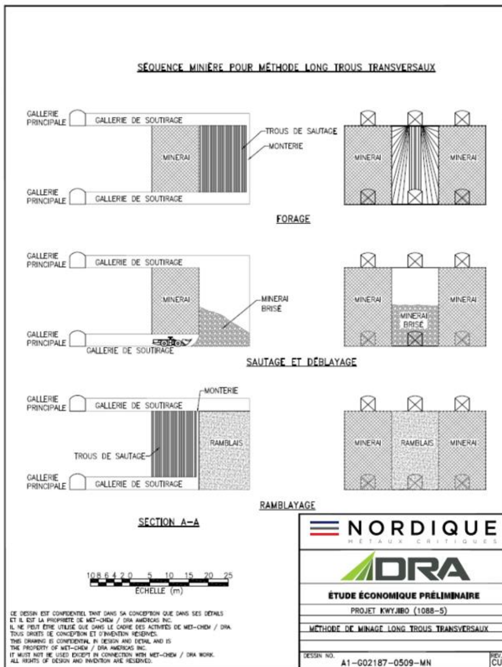
Figure 16.2 – Méthode de longs trous transversaux
