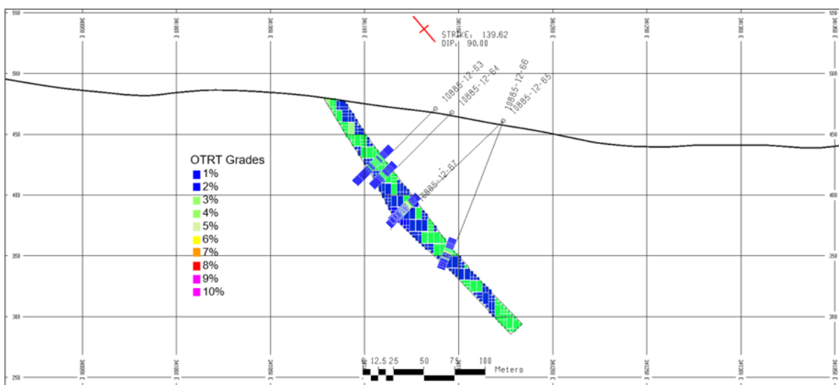
Figure 14.11 – Vue 2D d’une section type sur la Zone Nord Est
