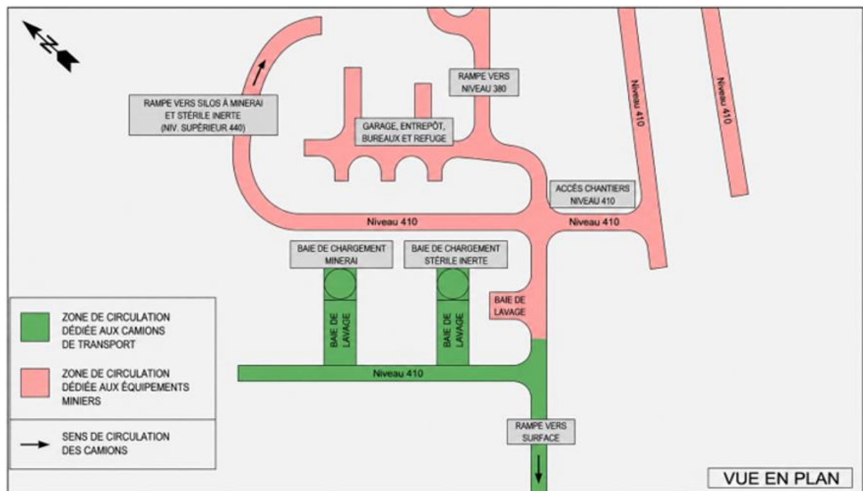
Figure 18.3 – Emplacement des baies de lavage
