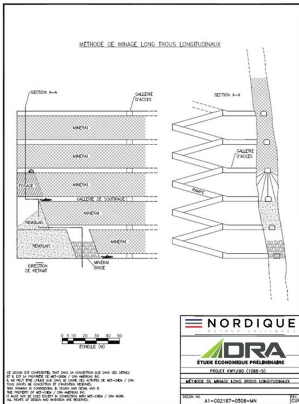
Figure 16.4 – Méthode typique d'exploitation par longs trous longitudinaux
