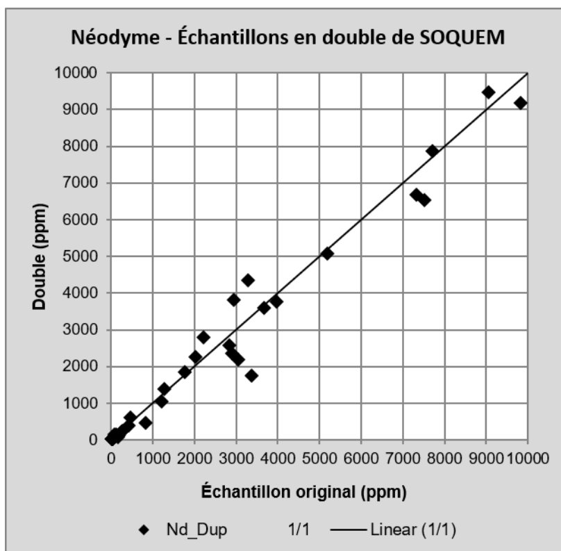
Figure 12.3 – Analyses originales et double pour le Néodyme
