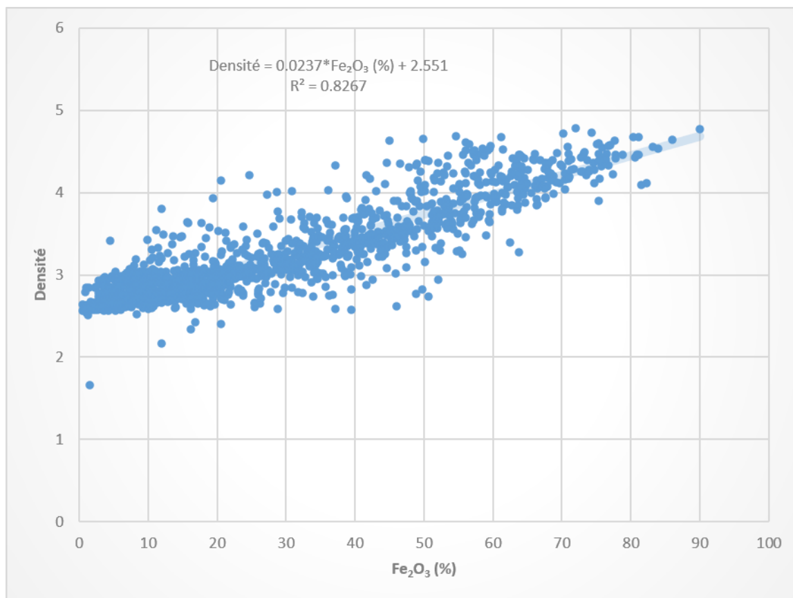
Figure 14.8 – Modèle régressif entre la densité et le \text{Fe}_2\text{O}_3 (%)
