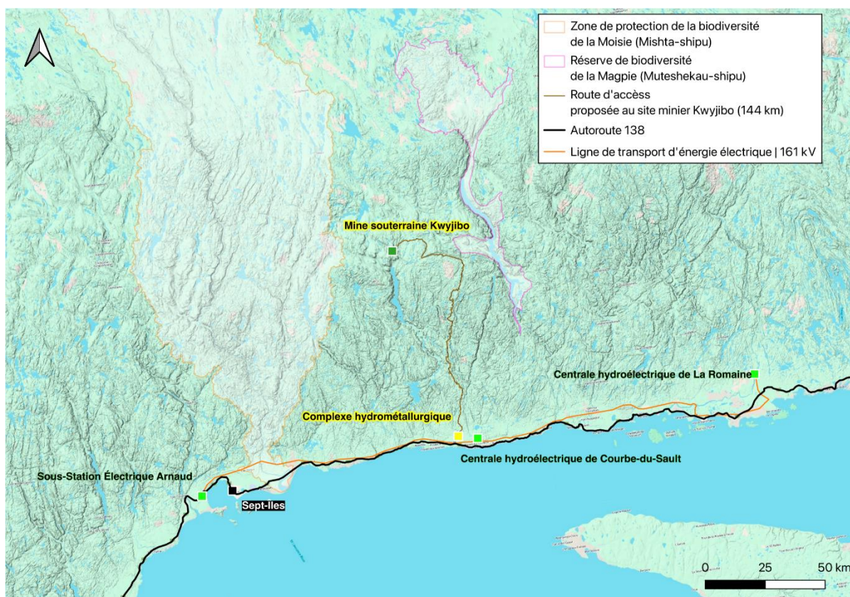
Figure 20.3 – Localisation du site minier Kwyjibo (2,67 ha), du complexe hydrométallurgique (19 ha) et du chemin d'accès reliant ces deux sites
