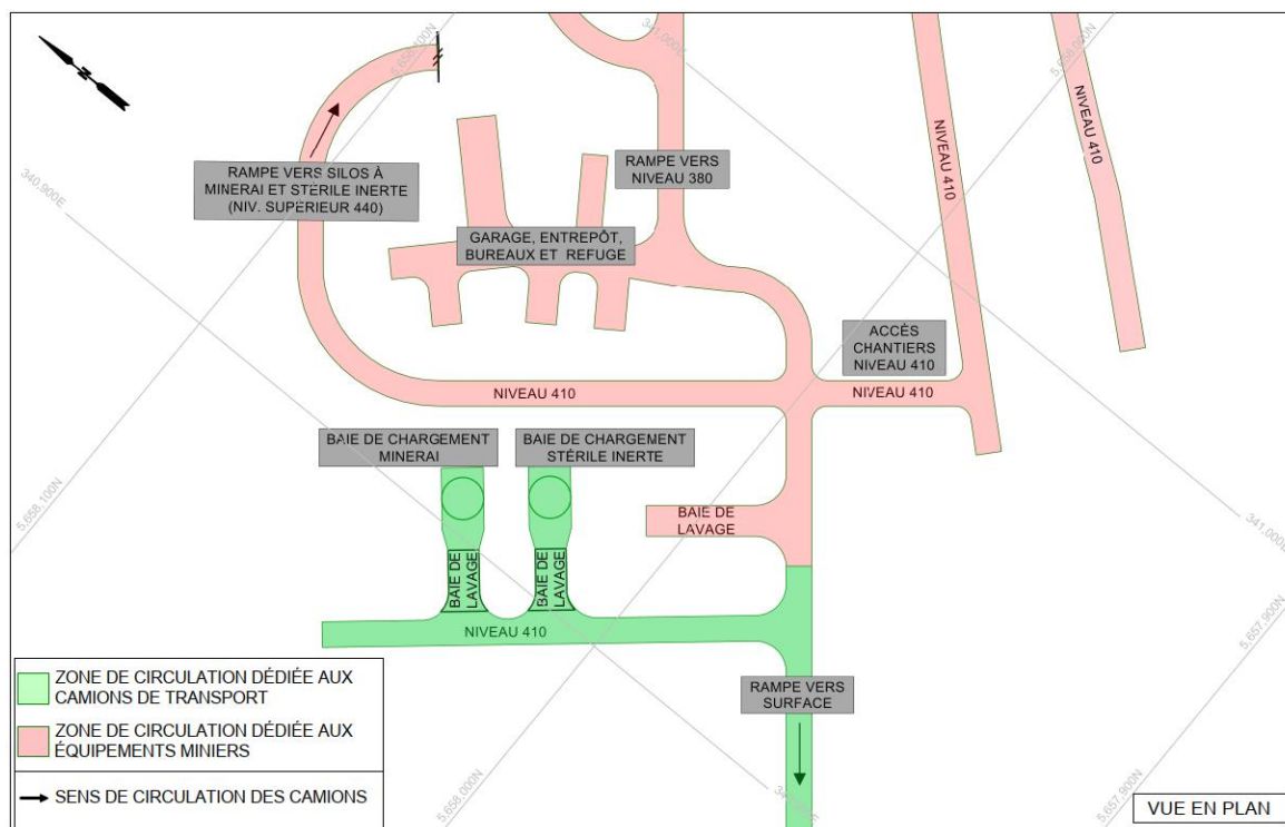
Figure 16.6 – Délimitation des zones de circulation et des aires de chargement, Niveau 410
