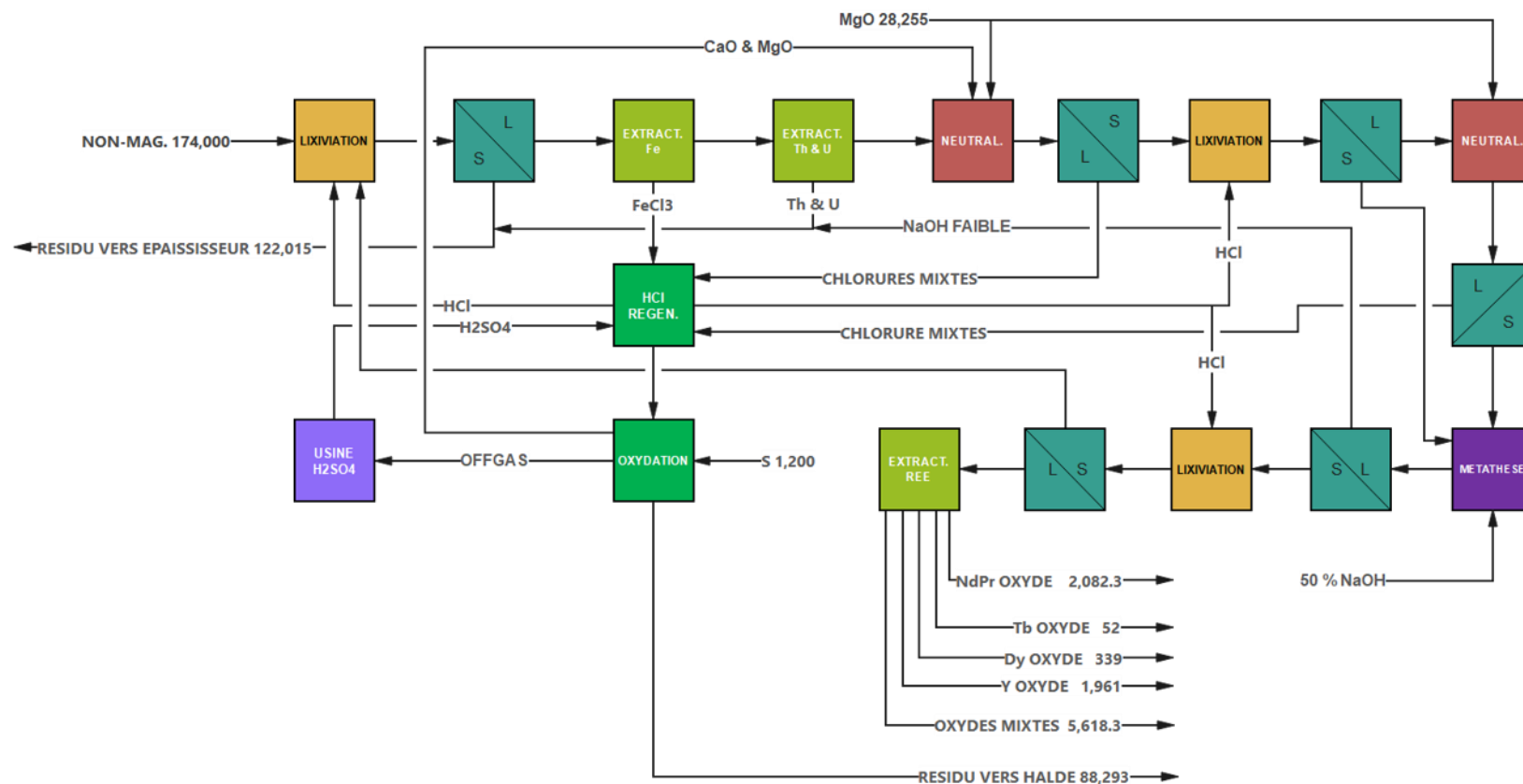
Figure 17.2 – Résumé du bilan de l'usine hydrométallurgique
