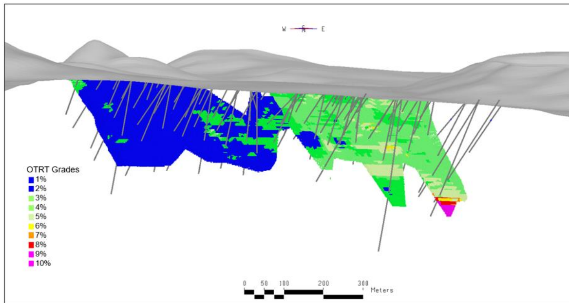
Figure 14.9 – Vue 3D (vers le Nord) du Modèle de Blocs de ressources
