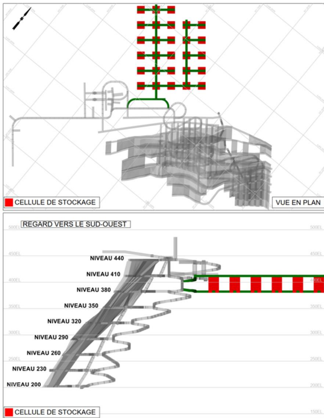
Figure 16.5– Agencement des cellules de stockage souterraines
