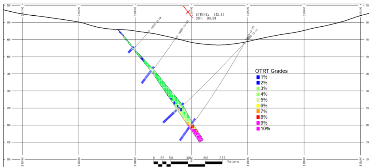
Figure 14.10 – Vue 2D d’une section type sur la Zone Nord Est
