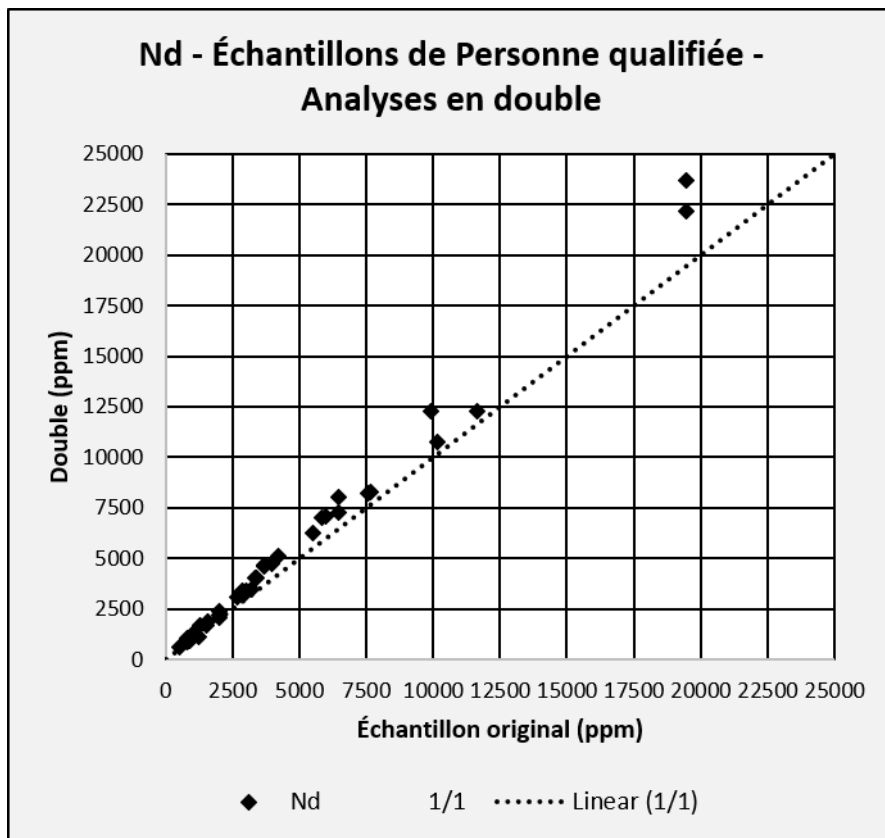
Figure 12.1 – Analyses du Néodyme dans les échantillons originaux et les doubles de DRA/Met-Chem
