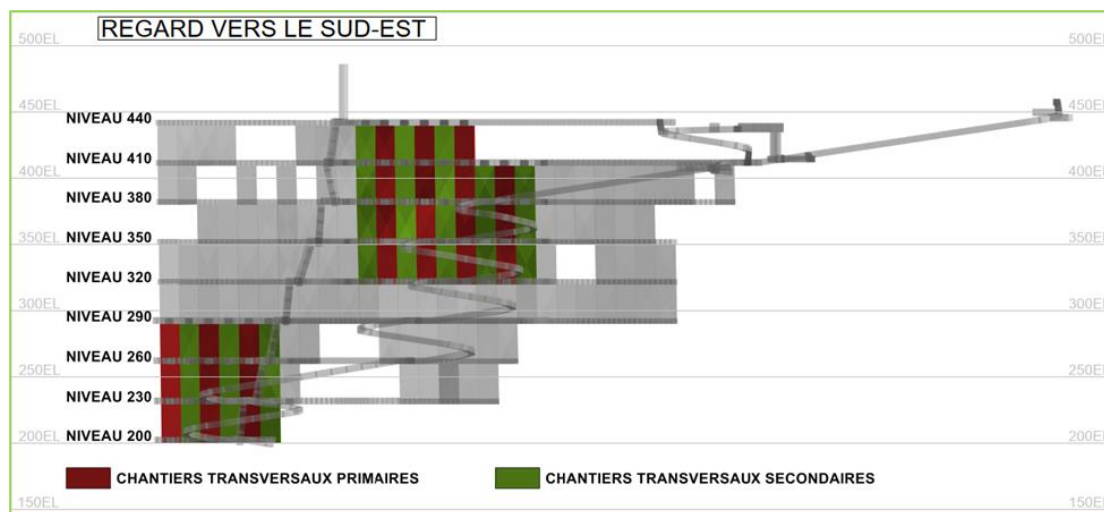
Figure 16.3 – Distribution des chantiers transversaux primaires et secondaires
