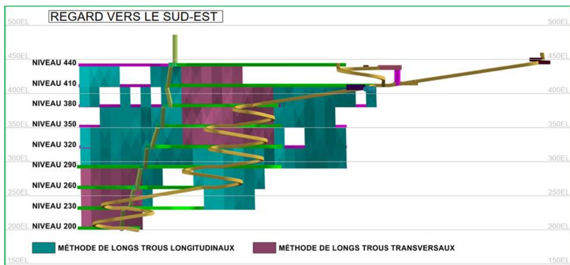
Figure 16.1 – Développement et chantiers de l'Horizon Josette
