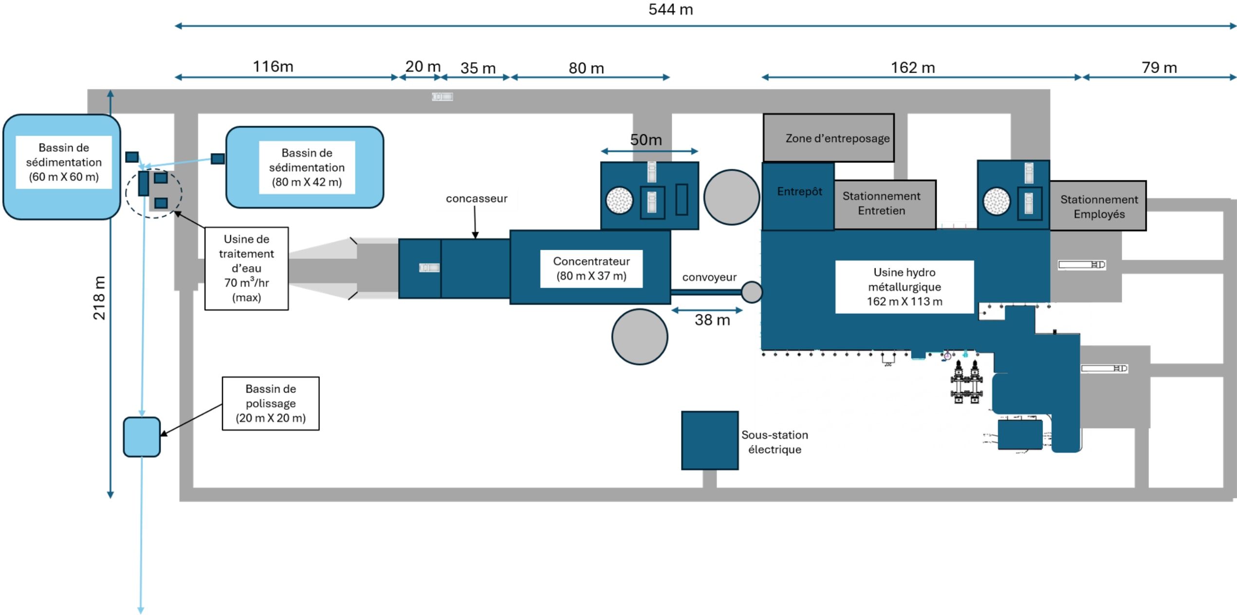
Figure 18.4 – Arrangement général du complexe hydrométallurgique
